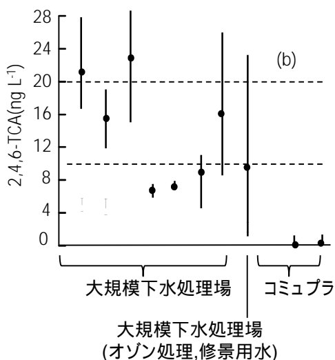
図 1(b) 下水処理水に含まれる 2,4,6-TCA
