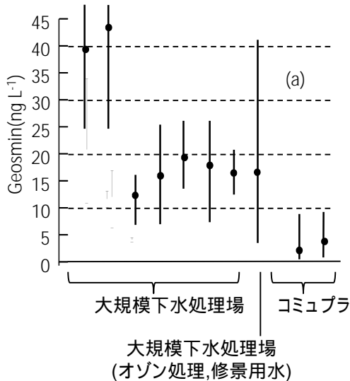
図 1(a) 下水処理水に含まれるジオスミン
