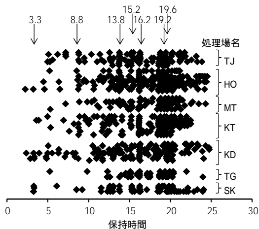
図3 におい嗅ぎ GC 測定におけるにおいを感じた GC 保持時間の一覧
