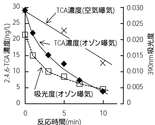
図 2 オゾン処理実験の結果
