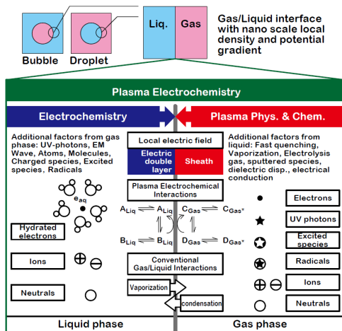
図3. 白藤らによる気液2層プラズマのコンセプト。新しい電気化学反応場と見なすことができる。
