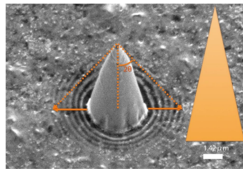
図6 .レーザー支援プラズマ CVD で作製したマイクロコーンの周囲に発達した波紋模様。図中のスケールバーは 1.42\mu\text{m} を示す。
