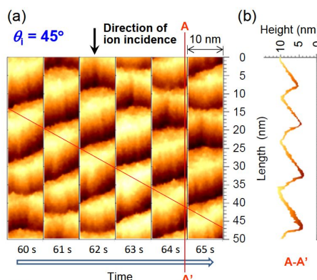
図5 .3次元原子スケールセルモデルによるエッチング表面でのラフネス形成の再現。
