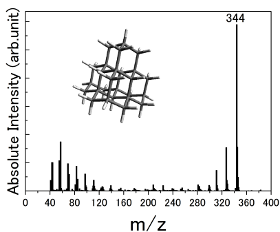
図2. 超臨界プラズマ反応場による高次ダイヤモンドドイドの合成。
