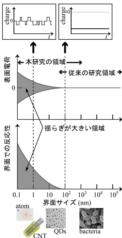
図1. 界面サイズがナノ領域になると様々な揺らぎが顕著になる。
