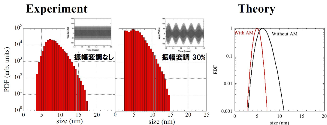
図4．プラズマ中ラジカル密度揺動によるナノ粒子サイズ分布の狭分散化（成長揺らぎの制御）。ナノ粒子成長とラジカルのカップリングを考慮に入れた理論計算結果は、実験結果とよく一致している。
