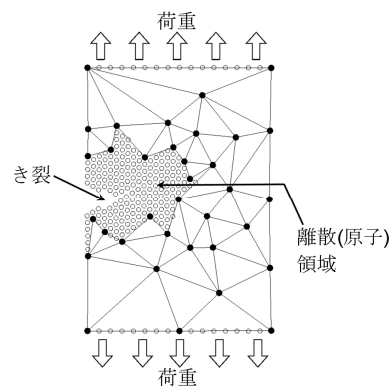
図 3 き裂先端の離散（原子）領域と要素領域
