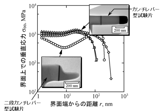
図 2 界面端近傍の応力分布
