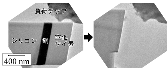
図 1 界面端からの破壊過程のその場観察像
