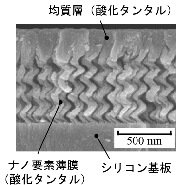
図4 ナノ要素薄膜
