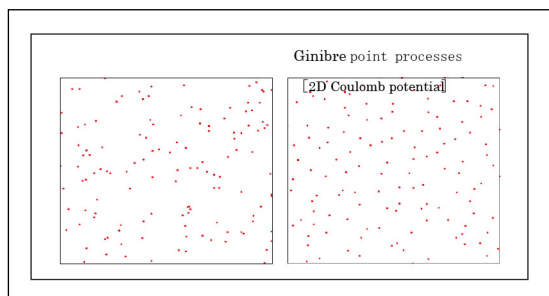
Poisson/Ginibre
