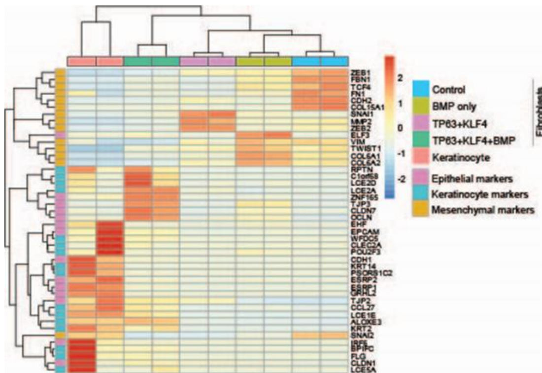
図2 BMP シグナル刺激による表皮細胞へのダイレクトリプログラミングの促進
