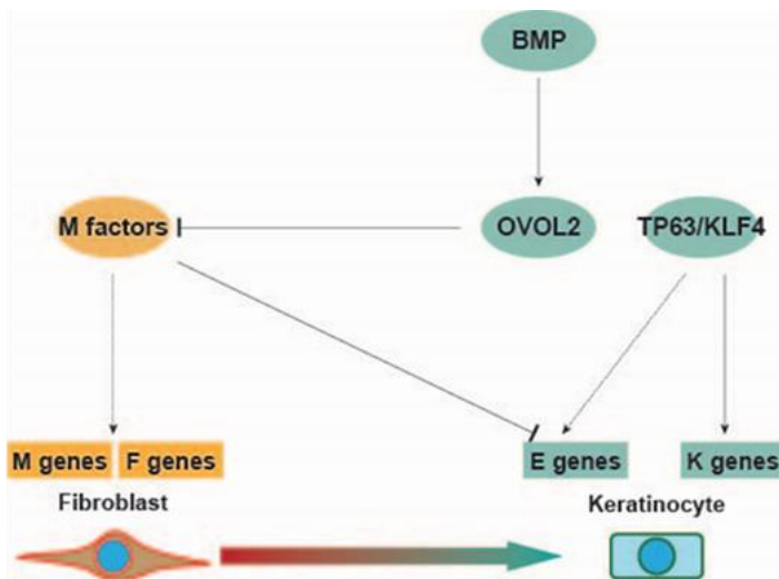
図1 線維芽細胞から表皮細胞への高効率ダイレクトリプログラミング法 OVOL2,TP63,KLF4 を用いた高効率ダイレクトリプログラミング法の図解
