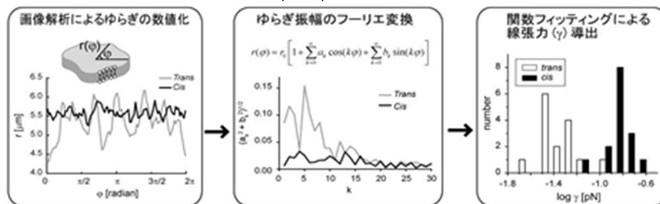
図1: 円盤膜の縁ゆらぎ解析による膜張力(γ)の導出。脂質構造変化とそれぞれの膜ゆらぎ挙動データを解析し、線張力を求めた例。
