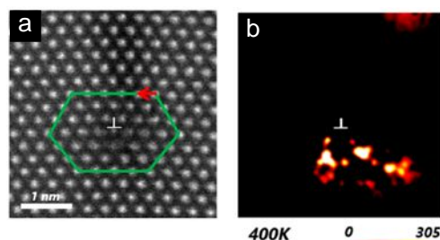
図3 (a)YSZ中の転位コアの原子像。(b)転位コア近傍におけるイオン伝導率(バルク比)。
