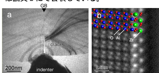
図2 (a)その場インデンテーション実験による粒界亀裂の形成。(b)粒界破面の原子像と理論構造モデル。
