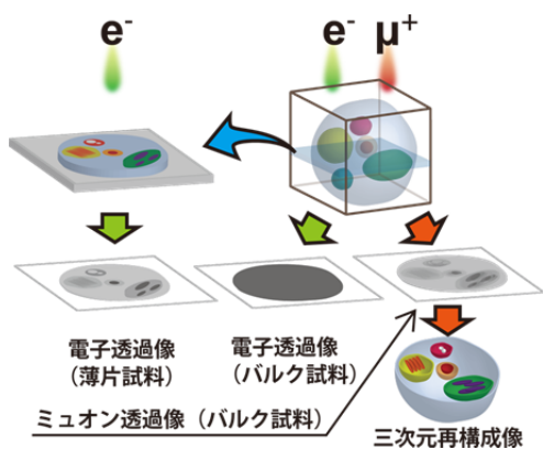
図 1. 透過型ミュオン顕微鏡が目指す、10 μm 厚試料の 3D イメージング vs. 電子顕微鏡。
