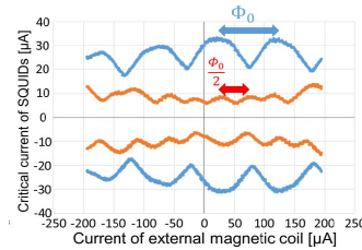
図 5 \pi - \pi - \pi SQUID の 2 並列化回路 (青) と通常の SQUID (橙) の臨界電流値の磁場応答特性
