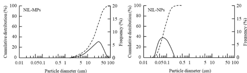
図 2 NIL-MPs (左) 及び NIL-NPs (中央) の粒子径分布と AFM イメージ (右)
