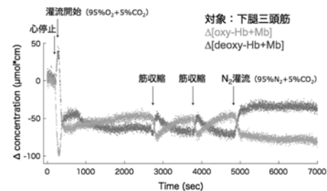
図1. 筋収縮開始直後からミオグロビン (Mb) の酸素解離が始まるのが明らかになった ( \Delta[oxy-] が低下し、 \Delta[deoxy-] が上昇)。
