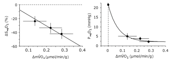
図2. 筋収縮の強度に応じて筋酸素摂取量 ( mVO_2 ) が上昇し、それと共に筋細胞内の Mb の酸素飽和度が低下した ( r^2=0.98 , p<0.01 )。また、Mb の酸素解離とともに、細胞内酸素濃度は急進的に低下し、 mVO_2 に応じて緩やかに低下した。
