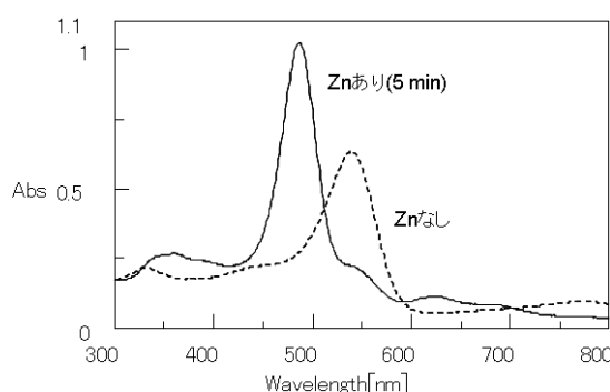
図 2. Zn 添加による OBTPyP の吸収スペクトル変化
