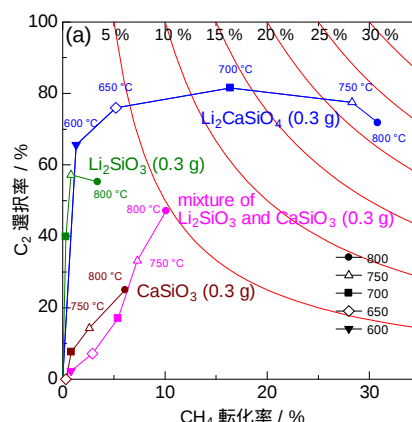
図 7. Li-Si または Ca-Si 系酸化物の OCM 触媒活性。
