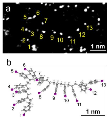
図3 (a)P4IS 分子鎖の ADF-STEM 像. (b)(a)を基に推定した P4IS 分子鎖立体構造.
