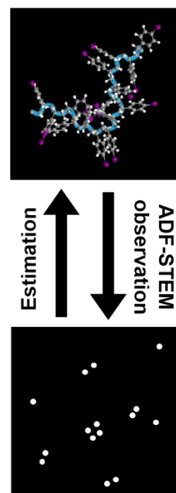
図1 ヨウ素修飾高分子の ADF-STEM 観察および構造推定の模式図。
