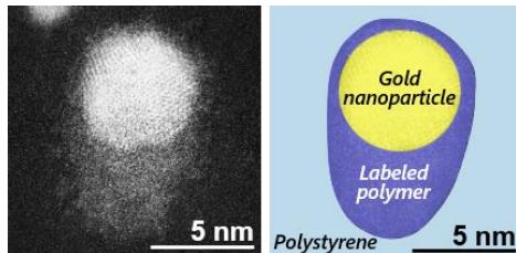
図4 金ナノ粒子に P4IS 分子鎖が吸着した構造の ADF-STEM 像および模式図.
