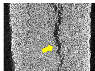
図4 CT画像断面(せん断帯)
