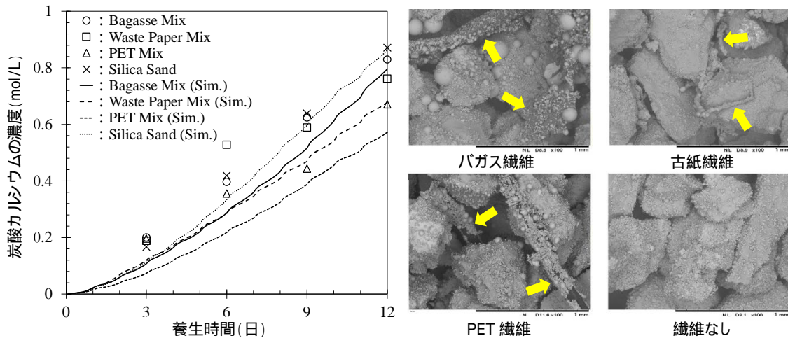
図2 解析結果と実験値の比較 (左図), 繊維材周りに析出する炭酸カルシウムの様子 (矢印は繊維材)
