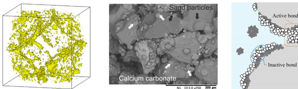
図5 シミュレーション結果の定性比較とメカニズム(左:炭酸カルシウムの析出解，中:炭酸カルシウムの析出実験の様子，右:粒子表面におけるアクティブボンド)
