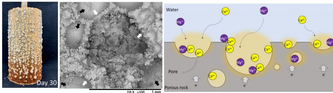
図3 多孔質岩モデルにおける電着物の析出 (左: 外観, 中: 微細構造 (白矢印が電着物), 右: イオン吸着機構)
