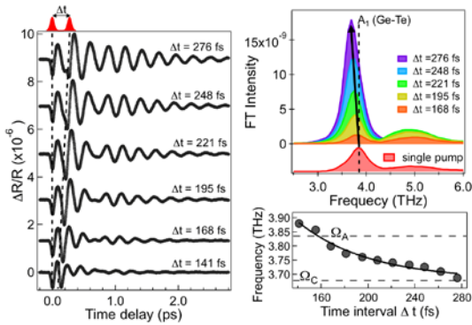
図 3. コヒーレント A_1 モードのパルス間隔( \Delta t )依存性(左). 右上図はフーリエ返還スペクトル、右下図はフーリエ変換スペクトルから得られた A_1 モードピーク周波数の \Delta t 依存性.
