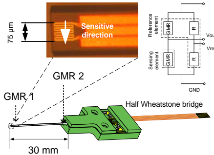
(b) 小形針状磁気プローブ
