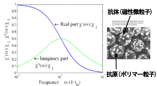
図7 磁気的免疫学的検査法における磁化特性
