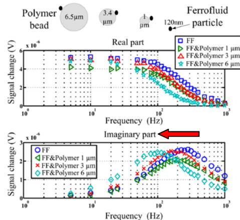
図12 ポリマーのサイズによる磁化率の周波数特性
