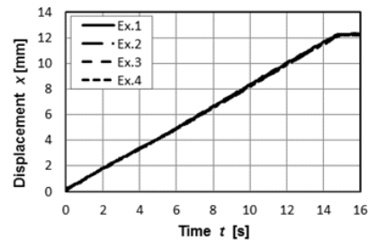
図11 アクチュエータの変位駆動 (周波数 f=400\text{Hz} )
