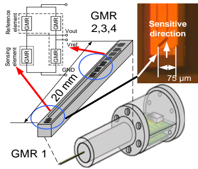
(a) 針状磁気プローブ(アンプボックス付)
