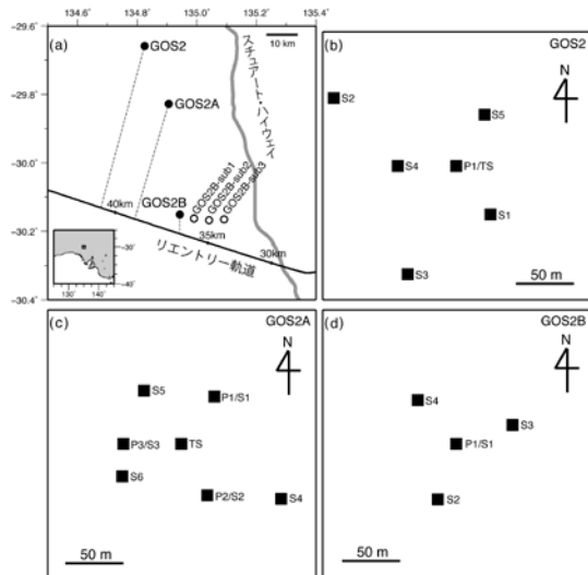
図 1. インフラサウンドセンサ/地震計の観測点分布。黒丸はアレイ観測点、白丸は地震計の単独観測点を表す。リエントリー軌道に沿って「はやぶさ」カプセルの飛行高度が記されている。(b) GOS2、(c) GOS2A、(d) GOS2Bのアレイ配置。Pはインフラサウンドセンサ、TSは三成分地震計、Sは鉛直成分地震計を表す。
