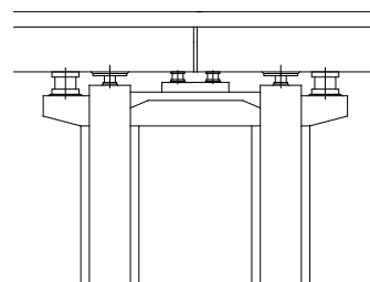
図-6 立体ラーメン橋台
