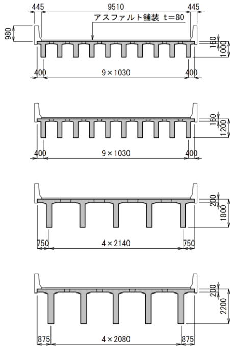
図-3 各解析モデルの断面形状 (上から支間長 20, 24, 30, 40m モデル)
