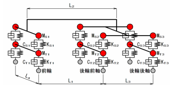
図-4 車両モデル
