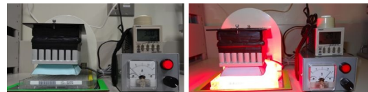
図1 . 96 ウェル治療用 LED 光照射システム
