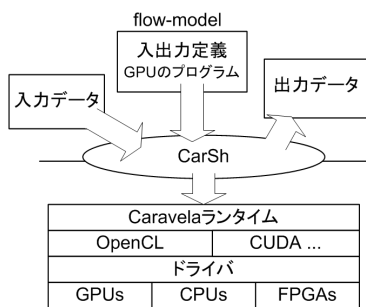
図 2 : CarSh のシステム構成
