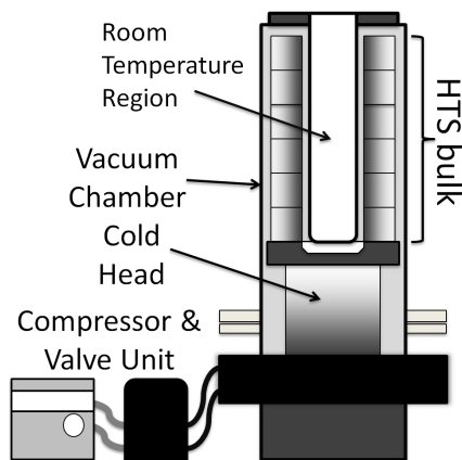
図2 クライオスタットの構造
