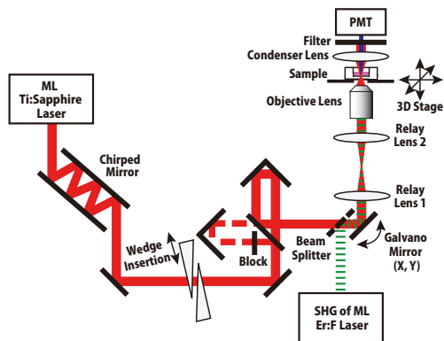
図 5 高感度 SHG 顕微鏡
