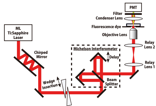
図3 2光子蛍光 (TPEF) 自己相関計
