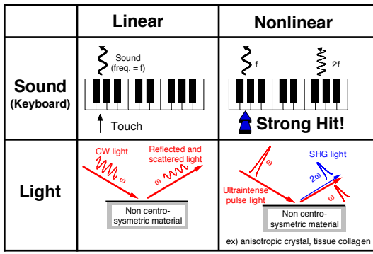
図1 SHG 光の原理
