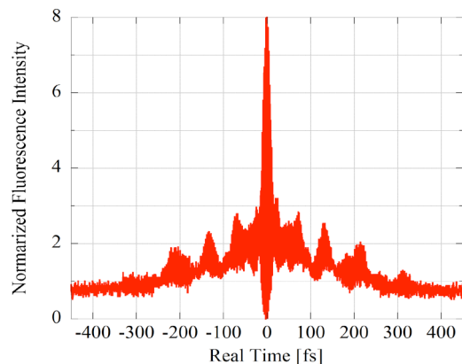
図4 焦点位置における自己相関波形
