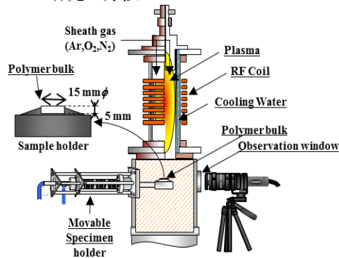
図1 ICTP 装置図
