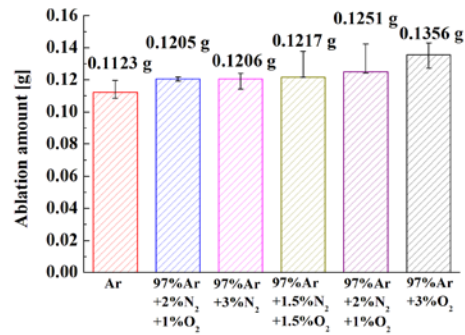
図4 熱プラズマ照射時のポリマーバルク材損耗量
