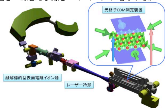
図1 レーザー冷却光格子EDM測定装置
