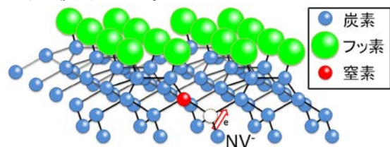
図2 フッ素末端 ダイヤモンド(001)2×1表面。フッ素原子は表面の不對電子を100%被覆可能である。
