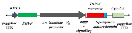
図 1. pBac-pvitellogenin-DsRed-GpDef の模式図
