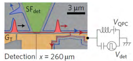
量子ホールカイラルエッジ状態におけるスピン電荷分離の検出素子(写真に色付け)
