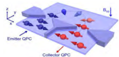
スピン軌道ロッキングによるスピン制御。磁気フォーカシングによりスピン生成・制御・検出を実現
