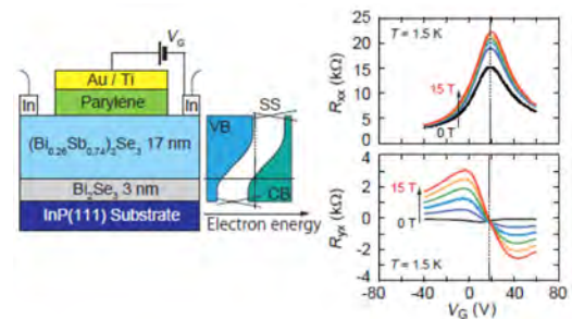
(\text{Bi}_{1-x}\text{Sb}_x)_2\text{Se}_3 をチャンネルとする電界効果トランジスタ. 縦・ホール抵抗のゲート電圧依存性
