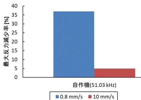
図3 ワイヤ型超音波振動子のスチレンフォームへの最大穿孔反力の超音波振動による減少率の穿孔速度間比較
