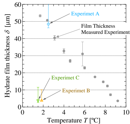
図 11 生成時水素レート膜厚と温度の関係
