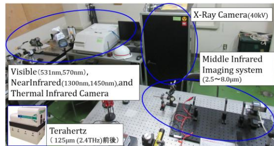
図2 開発した超広帯域スペクトル計測装置の外観(テラヘルツ計測装置は別室設置)。
