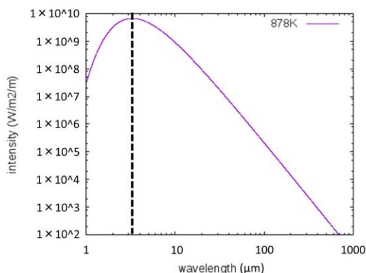
図4 セラミックヒーター温度特性計算結果.
