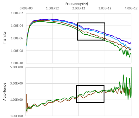
図10 テラヘルツ計測結果: パワースペクトル(上)(青と水色; 参照用ポリエチレン、茶; クヌギ枯葉、緑; アオキ生葉)、吸光度スペクトル(下)(緑; アオキ生葉、茶; アオキ枯葉)。
