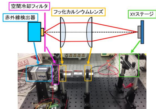
図3 開発した中間赤外域スペクトル計測装置.
