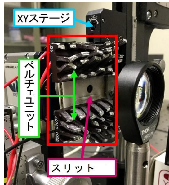
図5 空間冷却フィルタの外観.
