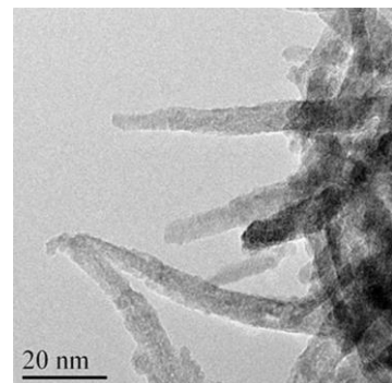
図1. 脱合金酸化により作製したナノロッド状セリア-ジルコニア固溶体のTEM像
