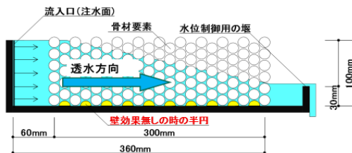
図-11 水平透水試験の MPS 法シミュレーションモデル (2次元)
