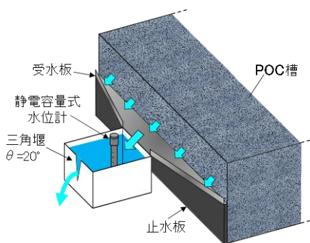
図-8 下流端における流量測定手法
