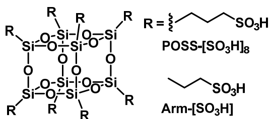
スキーム 1. POSS-[SO 3 H] 8 の化学構造。
