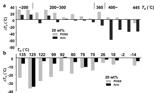
図 6. POSS-[SO 3 H] 8 添加時のイオン液体の (a) 熱分解温度と (b) 融点の変化。
