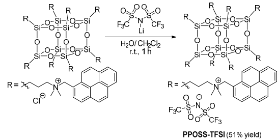
図 3. イオン性側鎖を有する修飾 POSS の合成.
