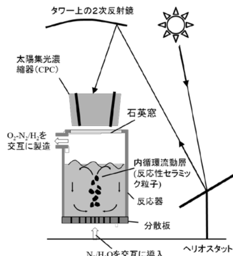
図1 流動層式ソーラー水分解器
