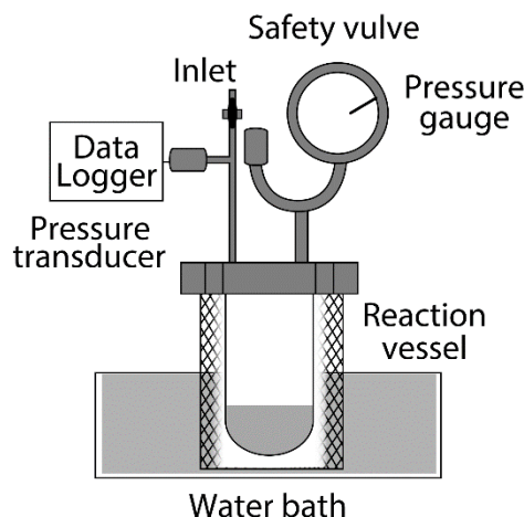
図1 反応熱量計装置概略図
