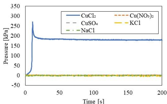
図2 \text{H}_2\text{O}_2 の圧力発生挙動
