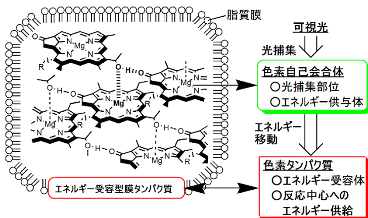
図1. 緑色硫黄光合成細菌の光捕集超分子複合体・クロロゾームの模式図.
