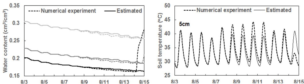
図8 8/8に取得した気象予測値を用いた土壌水分量と地温の計算値
