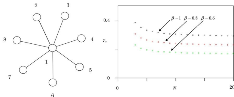
図2 スターグラフ（左）において感染が広がるかどうかの回復閾値（右）
