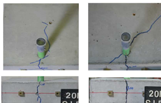
ひび割れ幅 1mm ひび割れ幅 3mm 図11 破砕剤充填後のひび割れの例
