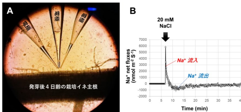
図1. 栽培イネの根の成熟領域表層のMIFE解析とNaCl刺激によるNa + 流出入の様子の例：A. MIFE測定開始直前の写真. B. 刺激前後のNa + の正味の流束
