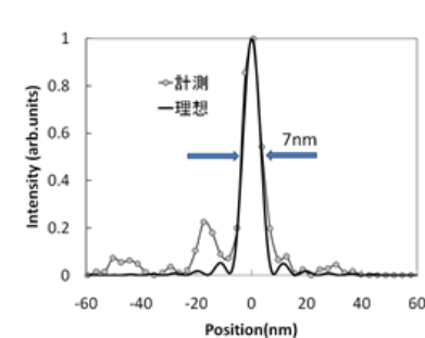
図 2 補償光学システムにより実現した世界最小の 7nm ビーム
