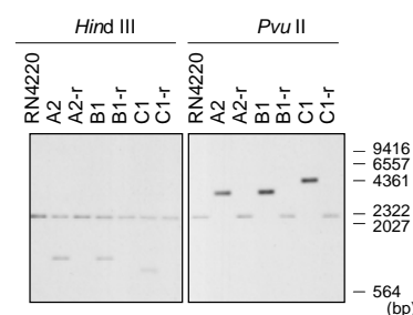
図3： sigH 遺伝子をプロベロブとしてサブザンブロット解析
