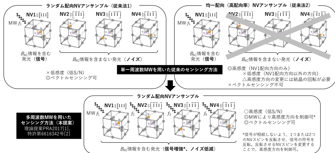
図 1. 単一周波数マイクロ波を用いた従来のベクトル磁場センシング方法と、本研究で提案する多周波数マイクロ波を用いた新規ベクトル磁場センシング方法の比較。
