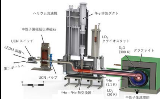
図1: TRIUMFに設置される超冷中性子源
