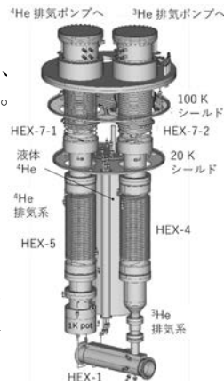
図 2: 冷凍機の内部構造
