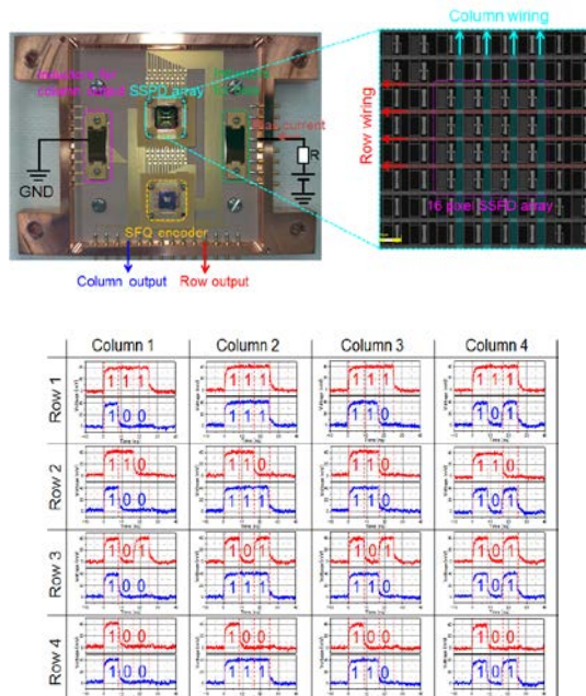
図2 SFQエンコーダを用いた行列読み出し方式4x4ピクセル SSPDアレイのチップ実装写真と出力波形 読み出し回路を設計・評価し、正常動作を確
