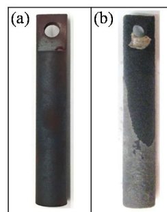
図4 加熱処理(1173 K-10 h)した3AL 試験片の外観 ((a)浸漬前、(b)Al-9Si-0.5Mg合金溶湯に9時間浸漬後に合金を除去)
