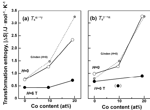
図2 Fe-Co合金の \alpha/\gamma 相変態における変態エントロピーのコバルト濃度依存性:○( H=0 ), ●( H=6T ). (a) \alpha \rightarrow \gamma 変態, (b) \gamma \rightarrow \alpha 変態
