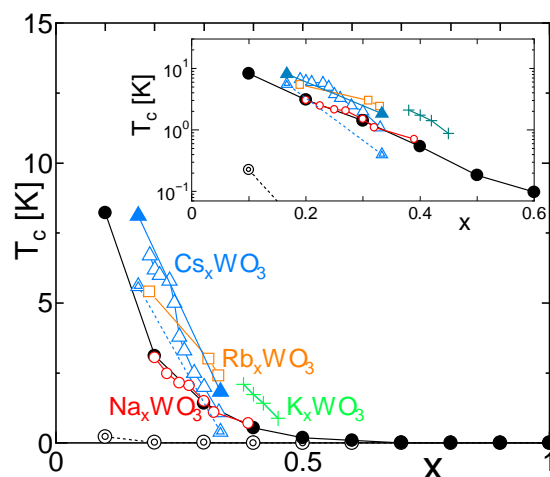
図 3: A_xWO_3 系における T_c の x 依存性
