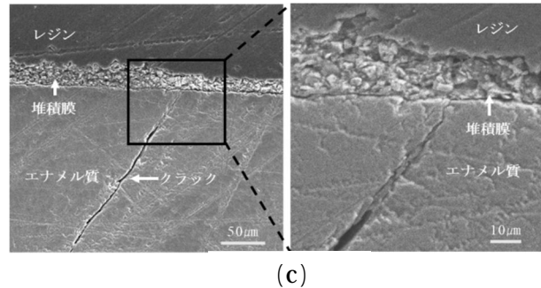
図 7. マイクロクラック修復結果
